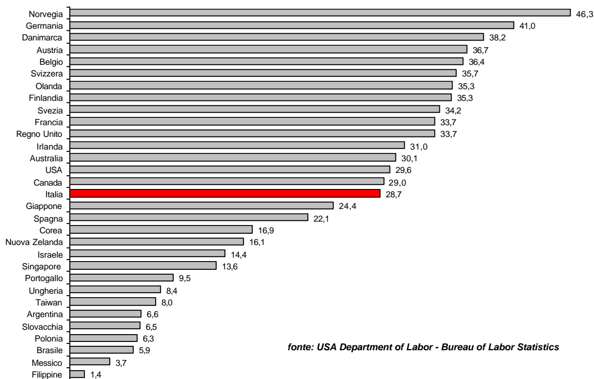
Graf. 2 - Costo orario del lavoro nel settore manifatturiero (tutti i lavoratori) nei diversi dei Paesi - 2006 (valori in dollari)
